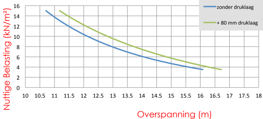
Overspanningsmogelijkheden FS400-1200
