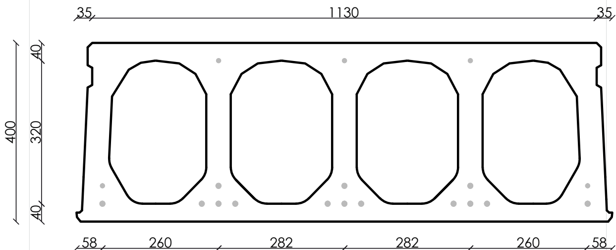
Overspanningsmogelijkheden FS400-1200
