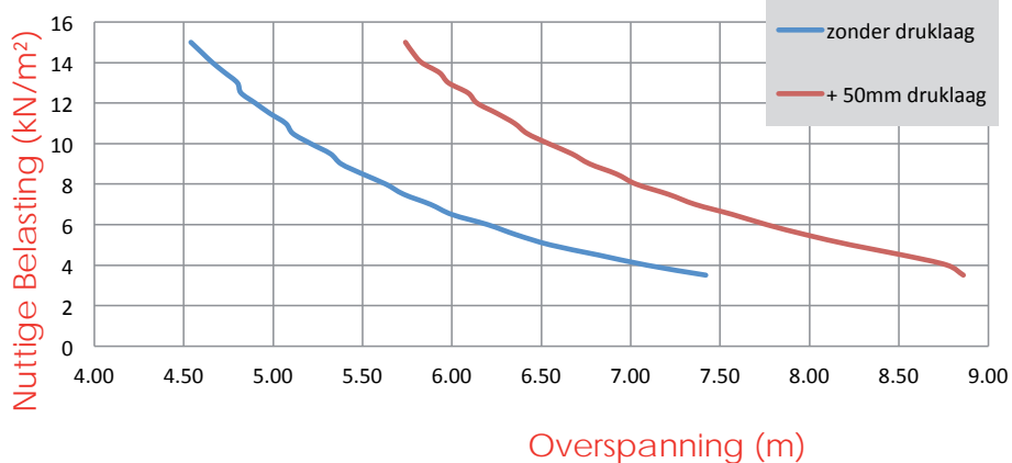
Overspanningsmogelijkheden FS180-600
